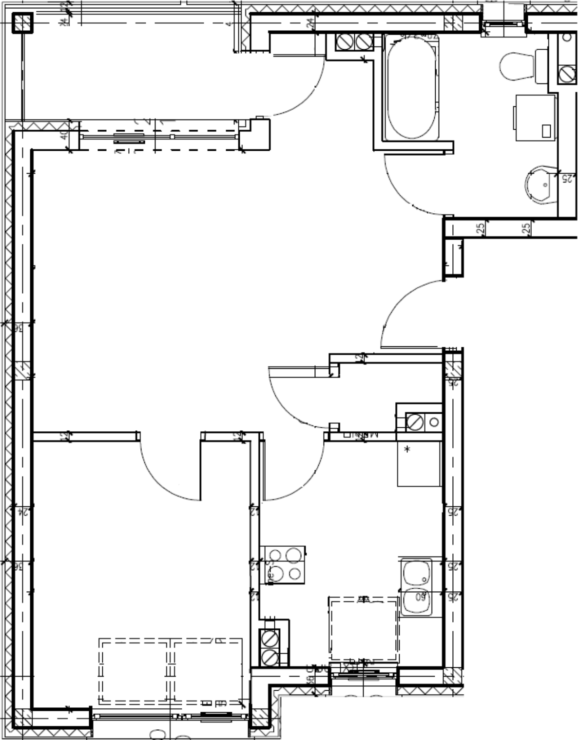
Rzut mieszkania przy ul. Wileńskiej 29 2 pokoje z kuchnią o pow. 43,02 m 2
